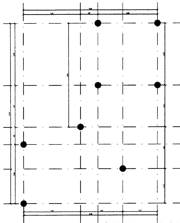
PLANTA LOCAÇÃO - CARAMANCHÃO Esc.: 1/25
